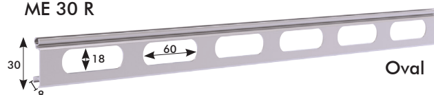
Kotelon mitoitus: Rullan ø D + 50 mm
